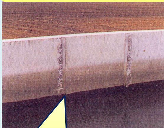
目地の損傷
