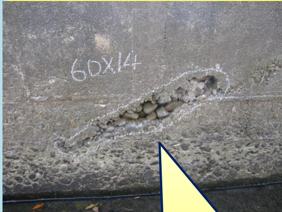
局所的な欠損
