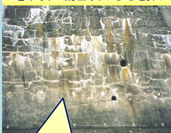
亀甲状・網目状のひび割れ
